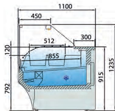
VE-10-RR ES
