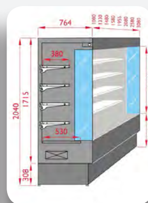
VULCANO C 80.
